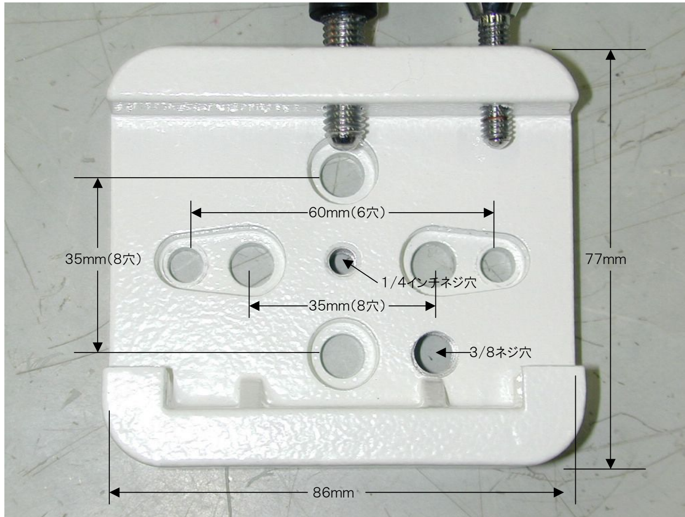
アリミゾベース寸法図
